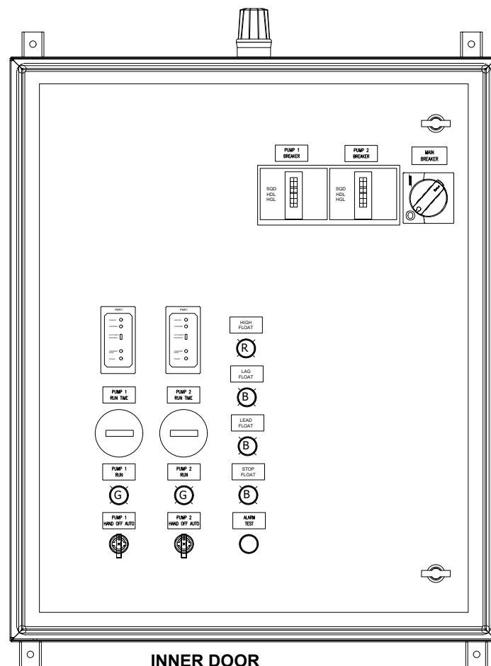
INNER DOOR
