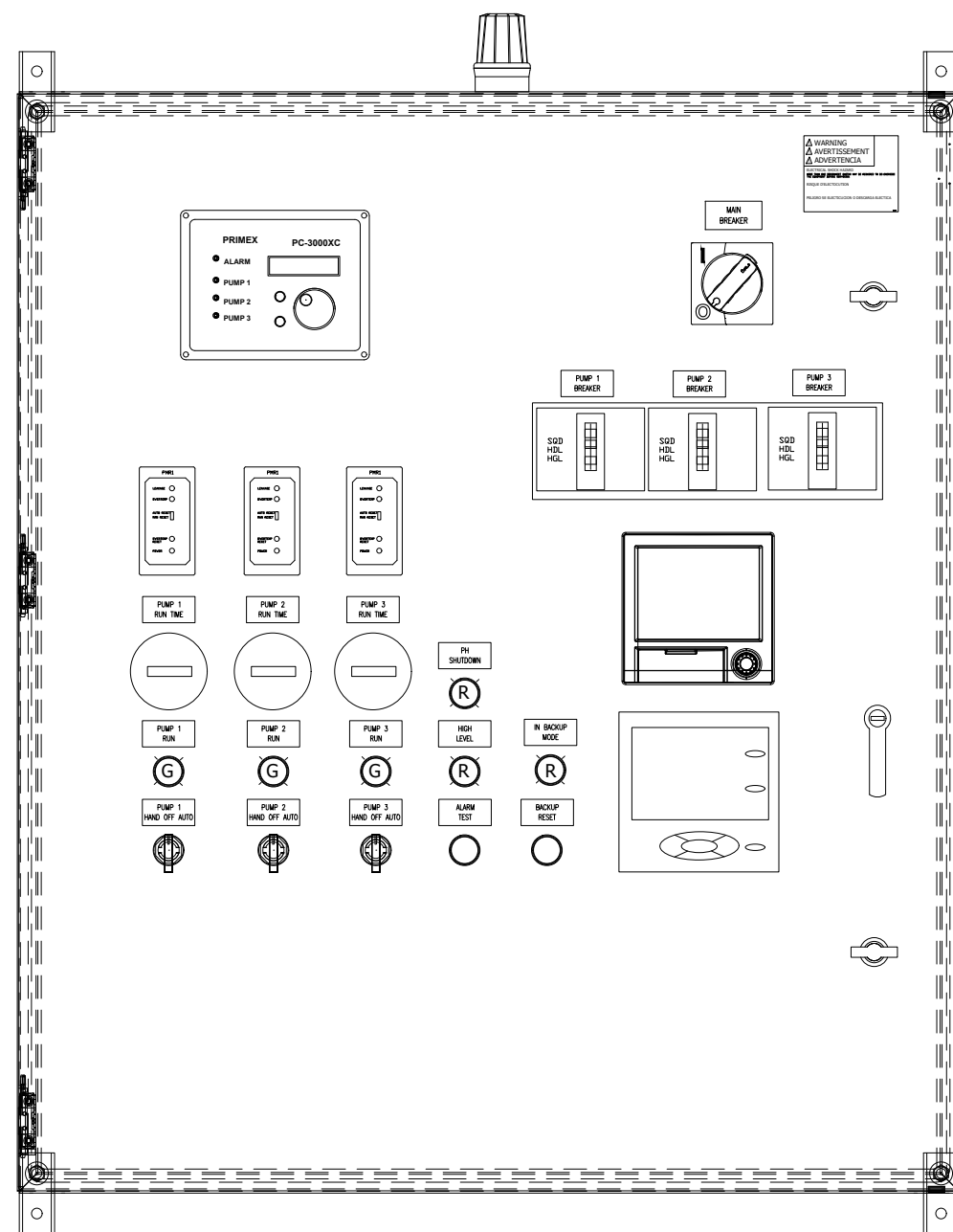
INNER DOOR
